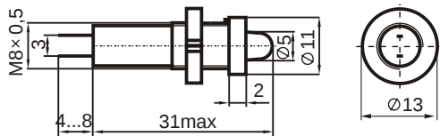
в пластмассовом корпусе
